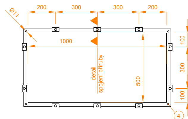
Obr. 10 Příruby zajištěné stahovacími svorkami
