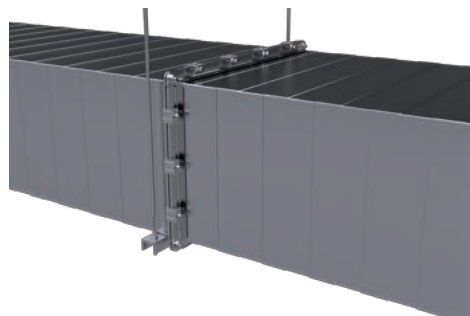
Obr. 62 Závěsné zařízení je možno s výhodou umísťovat do těsné blízkosti přírub
