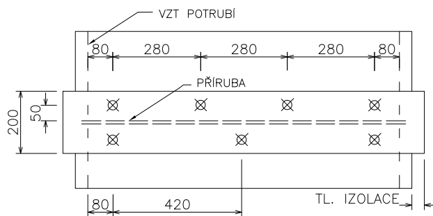
Obr. 20 Detail kotvení druhé vrstvy izolace, není-li zachováno krytí izolace nad přírubou min. tloušťky 20 mm
