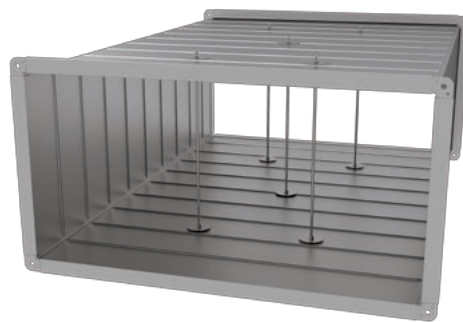
Obr. 57 Stanovení počtu výztuh pro potrubí 1000 x 500 mm, délka segmentu 1500 mm: (1 \times 1,5) \text{ m}^2 : 0,3 \text{ m}^2/\text{výztuha} = 5 výztuh rovnoměrně rozmístěných v ploše
