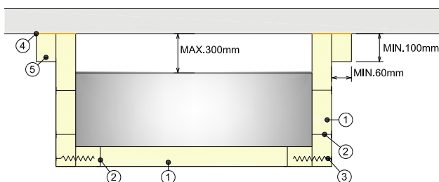
Obr. 76 Příčný řez svislým potrubím s izolací na 3 stranách
