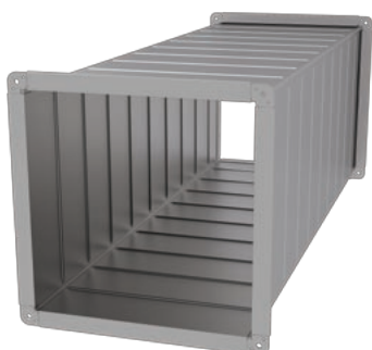
Obr. 56 Maximální rozměr potrubí, které se nevyztužuje, je 500 x 500 mm, délka segmentu 1500 mm
