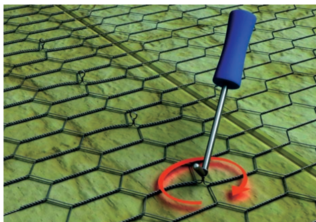
Obr. 54 Spojení rohoží překroucením přiléhajících okrajů pletiva do sebe po vzdálenosti cca 100 mm
