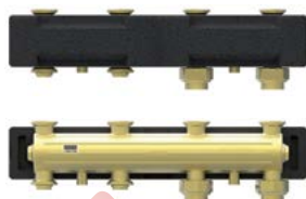
1 vstup / 2 okruhy
