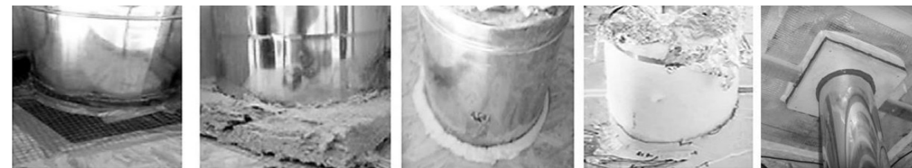
Obr. 2: ukázka řemeslného zpracování a utěsnění prostupu komínového tělesa střešní konstrukcí: a) vzduchotěsné utěsnění; b) utěsnění minerální vatou; c) vyplnění izolačním materiálem pro střechy; d) vyplnění PIR (2); e) průchod střechem za použití izolační průchodky
