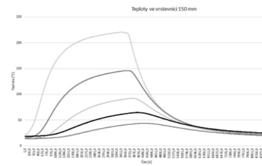
Obrázek 2.1 – povrchové teploty – průchodka vyplněna minerální izolací.
