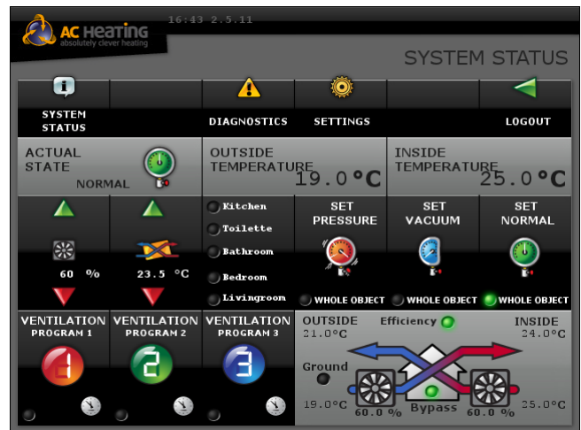
Obr. 14: Nastavení xCC Air (rekuperace)
